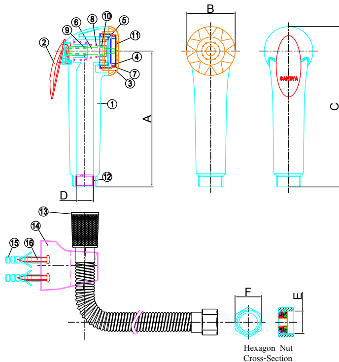
Dimension มิติ (mm.)
