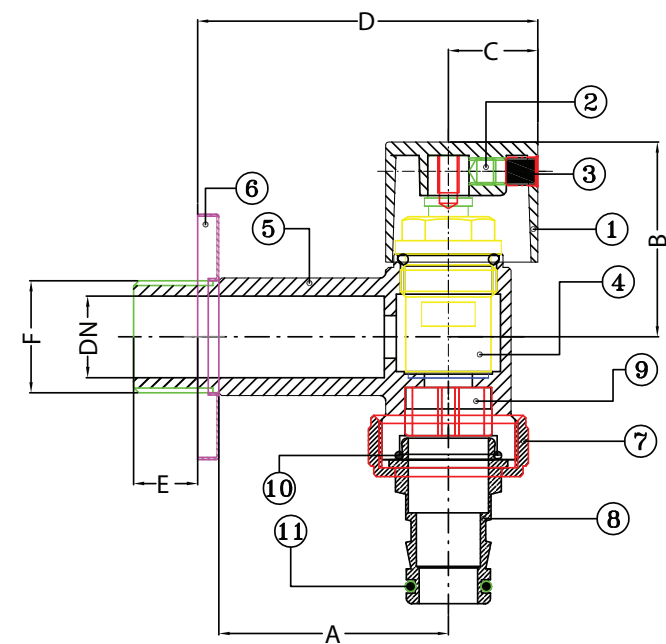
Dimension มิติ (mm.)
