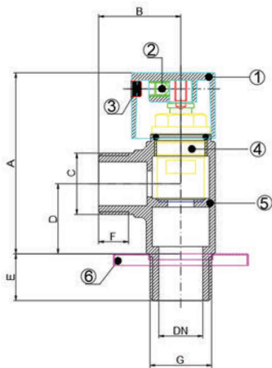
Dimension มิติ (mm.)
