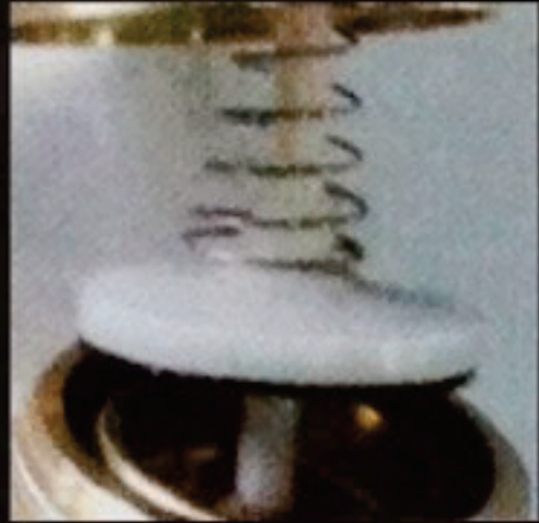
Durable Shaft made of Nylon สับ ทำจากไนลอนแท้ ทนทาน
